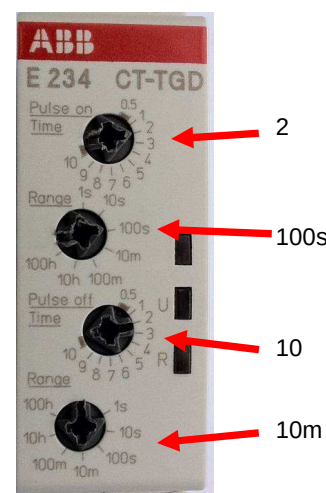
Minuterie de la pompe pour la recirculation des boues
